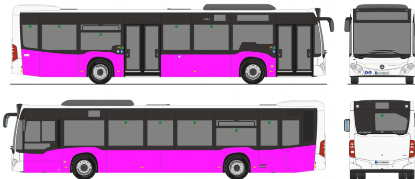
Rumpfbeschriftung beidseitig
